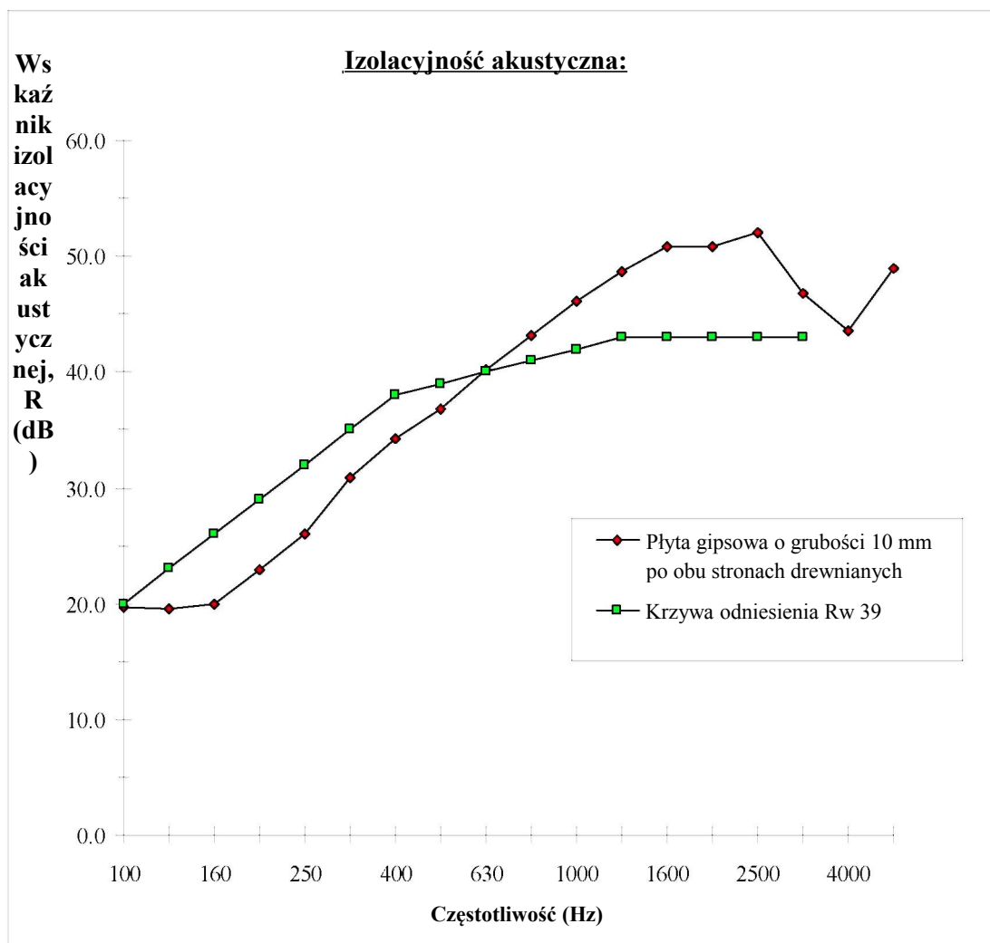
Wykres I: Tabela wyników dla płyty gipsowej o grubości 10 mm z drewnianą konstrukcją szkieletową 90 mm i izolacją piankową Selection 500.
